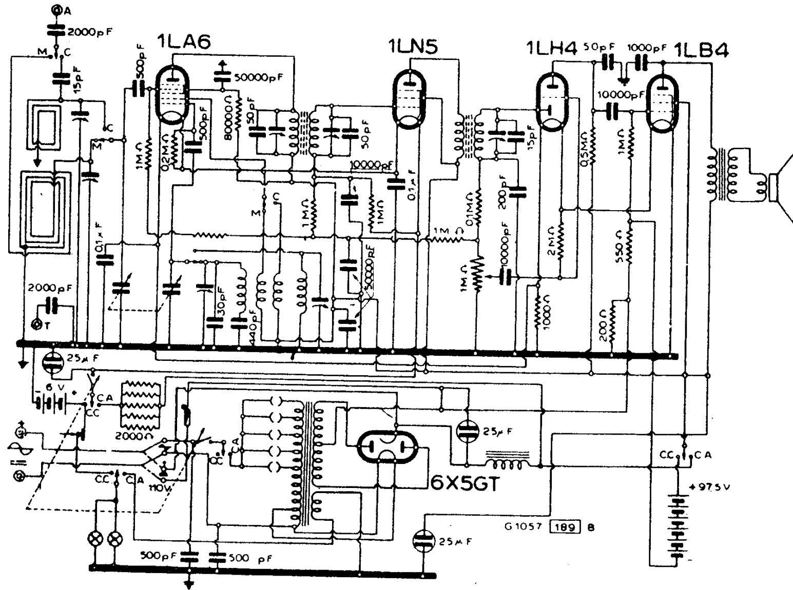
F.I.M.I. - MOD. PHONOLA « 545/1 »
